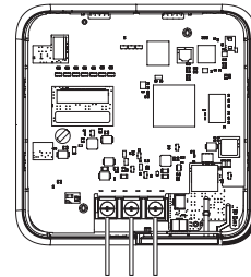
GND / SIG / 12V
