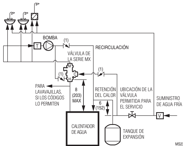
Fig. 4. Calentador con recirculación. Dimensiones expresadas en pulgadas (mm).
