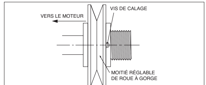
Figure 19.3 - Réglage de tension de la courroie
