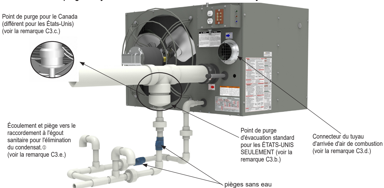
Figure 10.1 - Point de purge du système d'évacuation et raccords du tuyau d'écoulement
