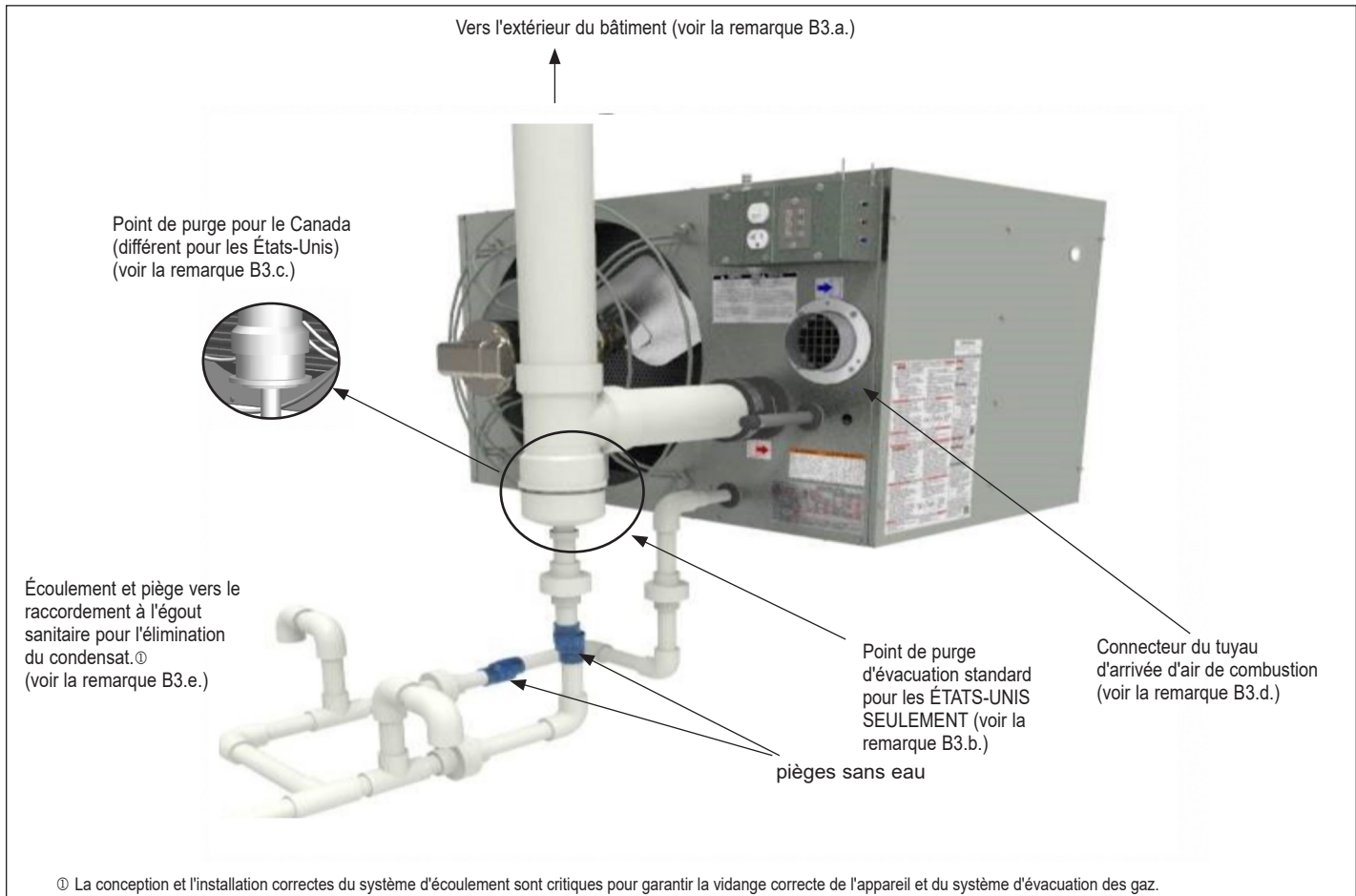
Figure 8.1 - Point de purge du système d'évacuation et raccords du tuyau d'écoulement
