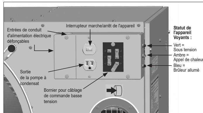
Figure 17.1 - Câblage d'alimentation/commande
