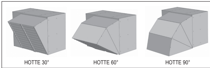
Figure 25.2 - Portée/couverture du sol avec hotte à 30° et 60°
