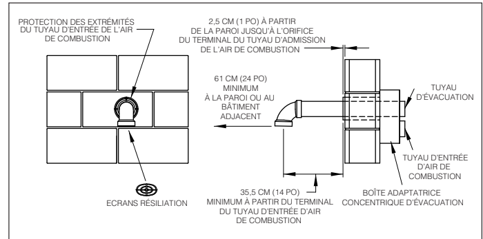
Figure 12.3 - Ensemble d'évacuation des gaz concentrique horizontale
