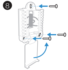
Utiliser les 3 vis no 8 de 1 1/2 po fournies
