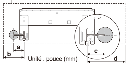
Cadre de l'unité intérieure
